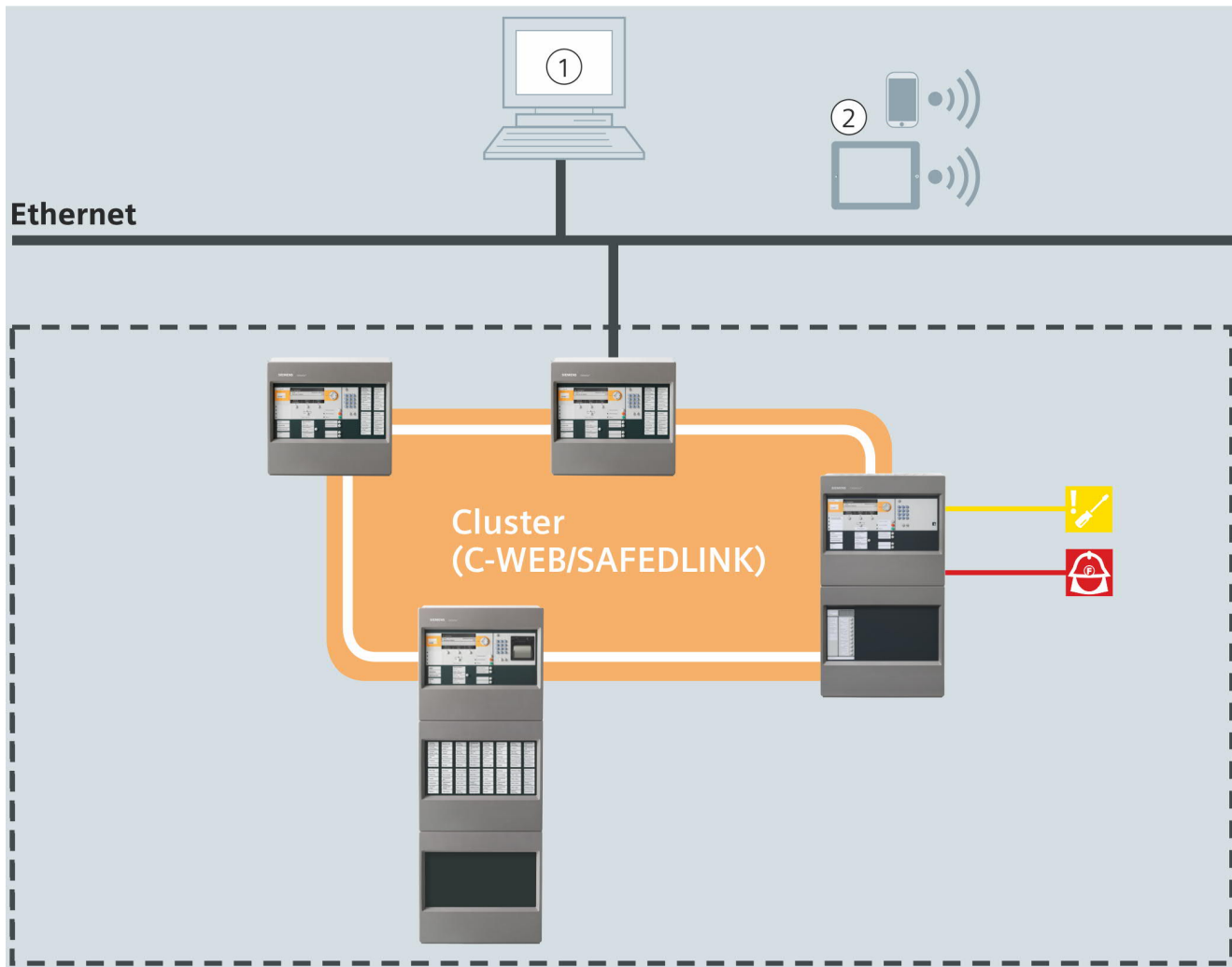
Fig. 2: Sub-net
