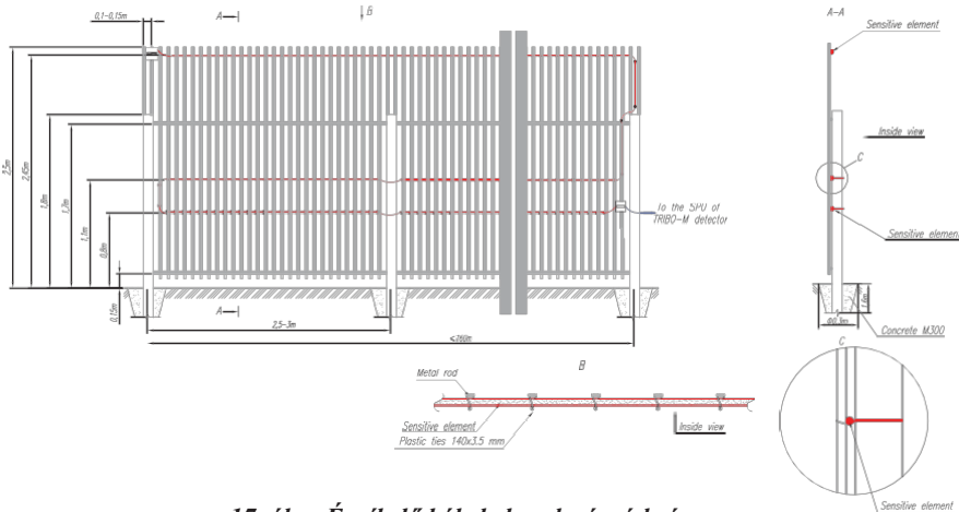
17. ábra Érzékelő kábel elrendezés rúd rácsra
