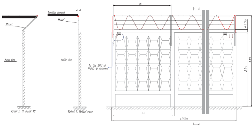
7. ábra Érzékelő kábel elrendezés szögeshálóra
