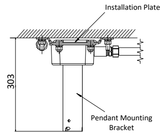
DS-1691ZJ-X Dimensions
