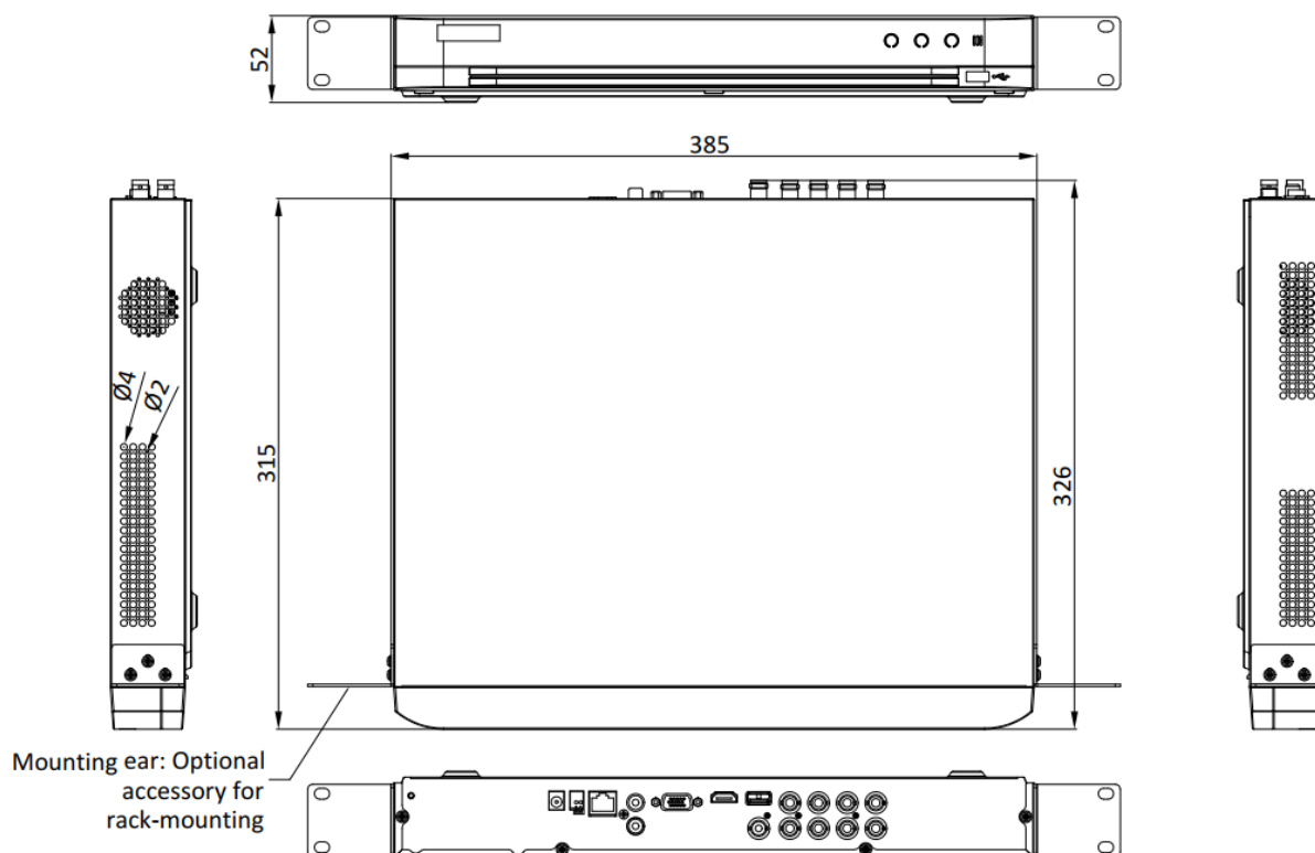
scale/1:1;Unit/mm
